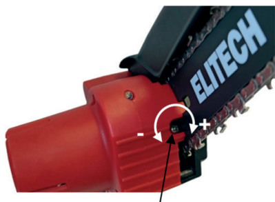
Шынжырды тарту бұрандасы 2-сурет
