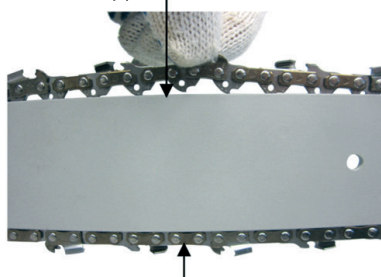
Шынжыр шинаға тығыз 3-сурет
