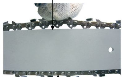
Շղթան սերտորեն տեղավորվում է անվադողի վրա
