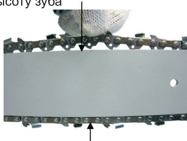
Цепь плотно прилегает к шине
