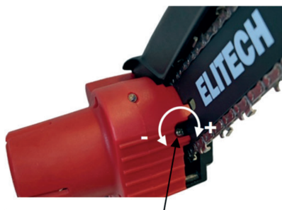
Винт натяжения цепи
