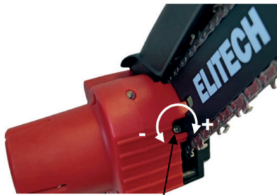
Շղթայի լարվածության պտուտակ
